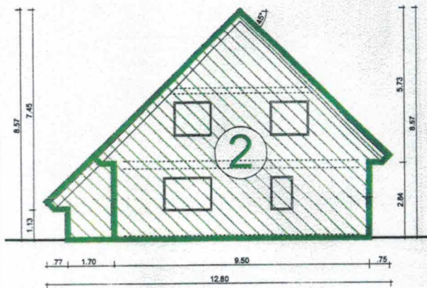
Ansicht Süd-Ost
