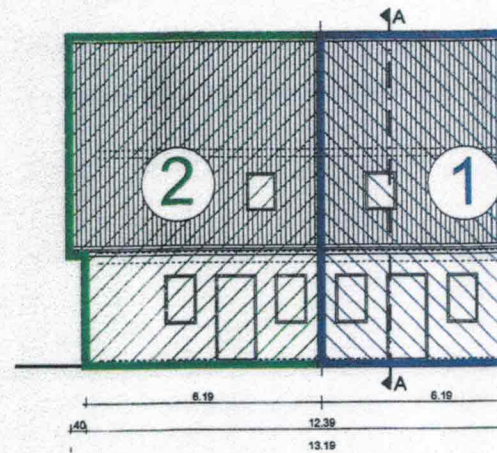
Ansicht Süd-West
