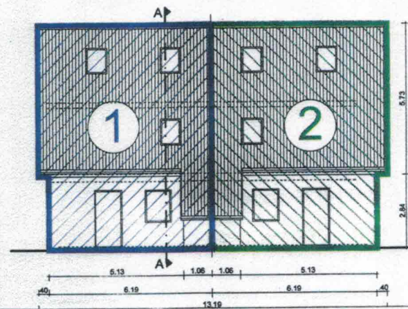
Ansicht Süd-West
