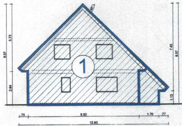
Ansicht Süd-Ost
