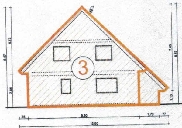
Ansicht Süd-Ost
