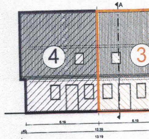
Ansicht Süd-West
