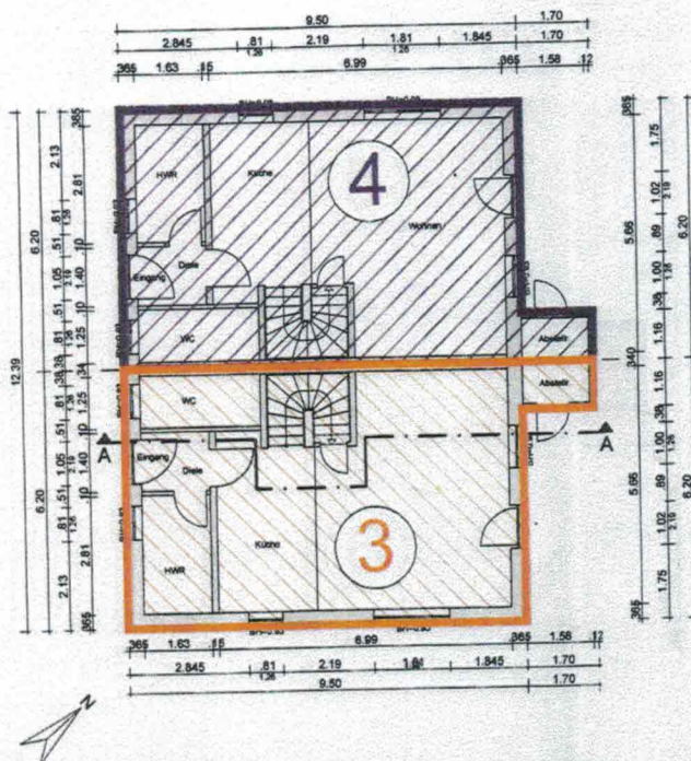
EG
