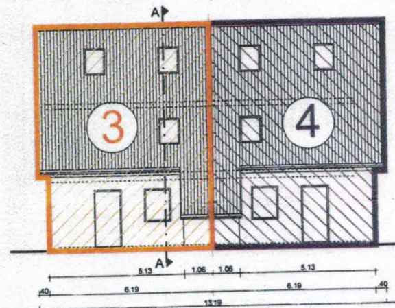
Ansicht Süd-West
