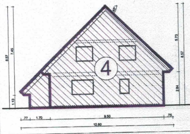
Ansicht Süd-Ost
