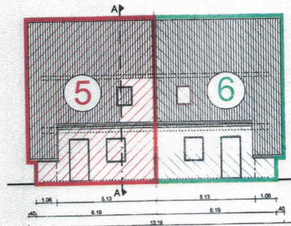
Ansicht Nord-Ost
