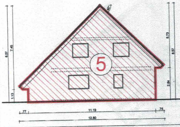
Ansicht Nord-West
