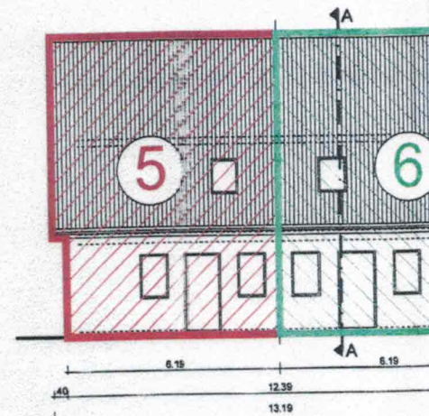
Ansicht Nord-Ost
