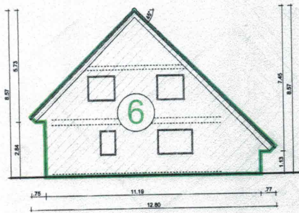
Ansicht Nord-West
