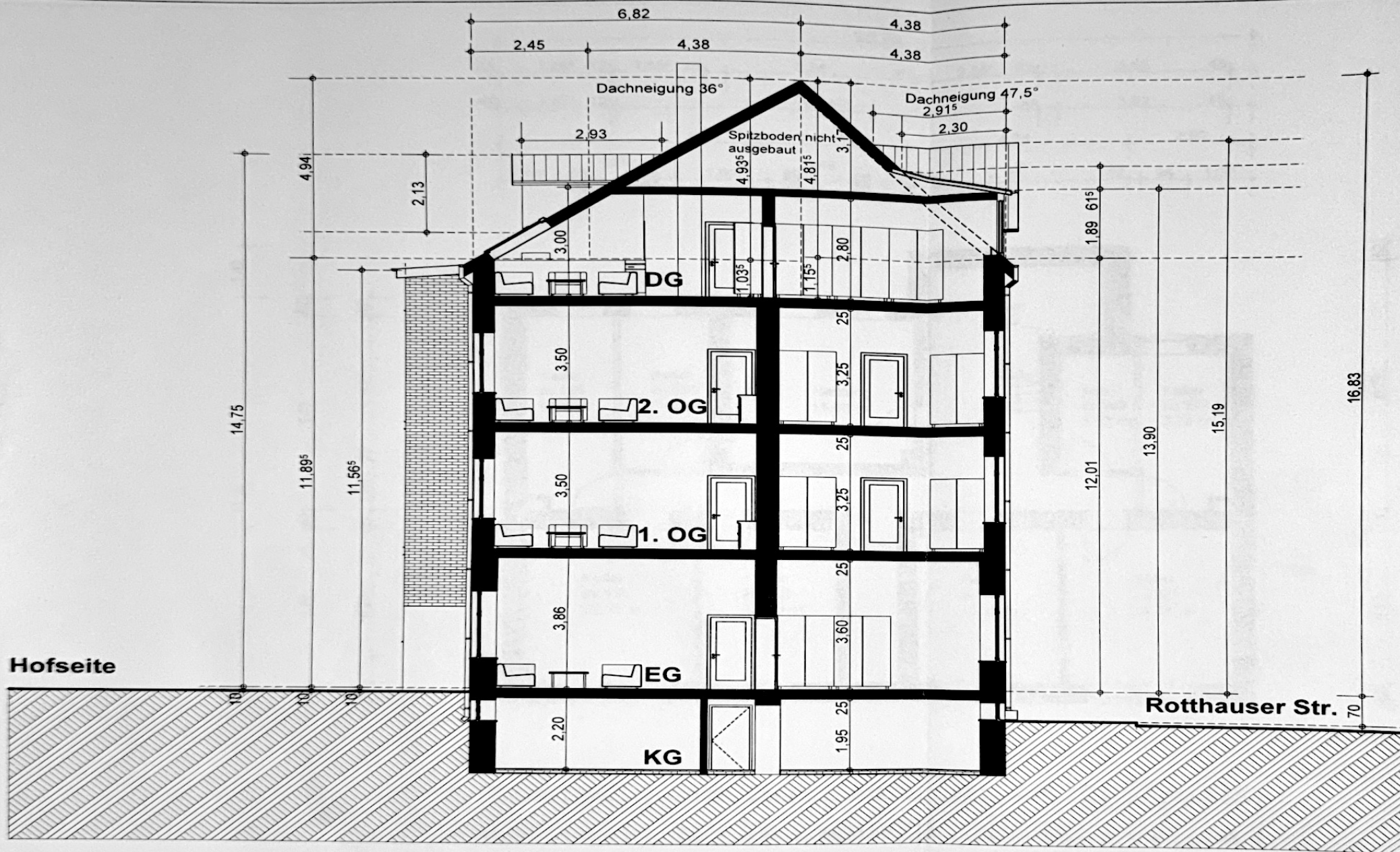
Schnitt A- A
