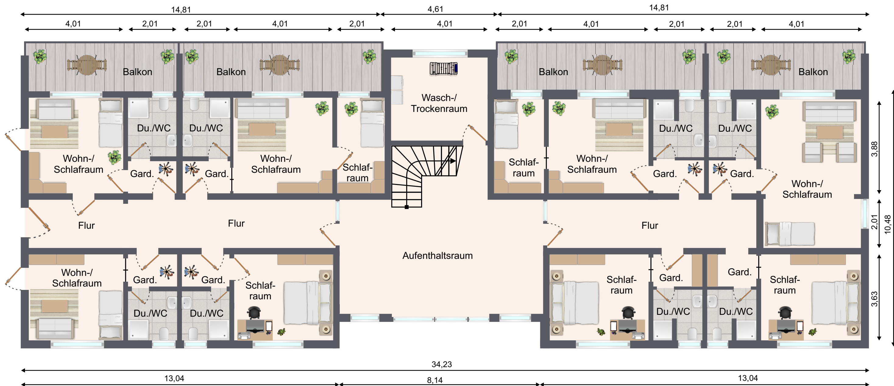
Obergeschoss Haupthaus
