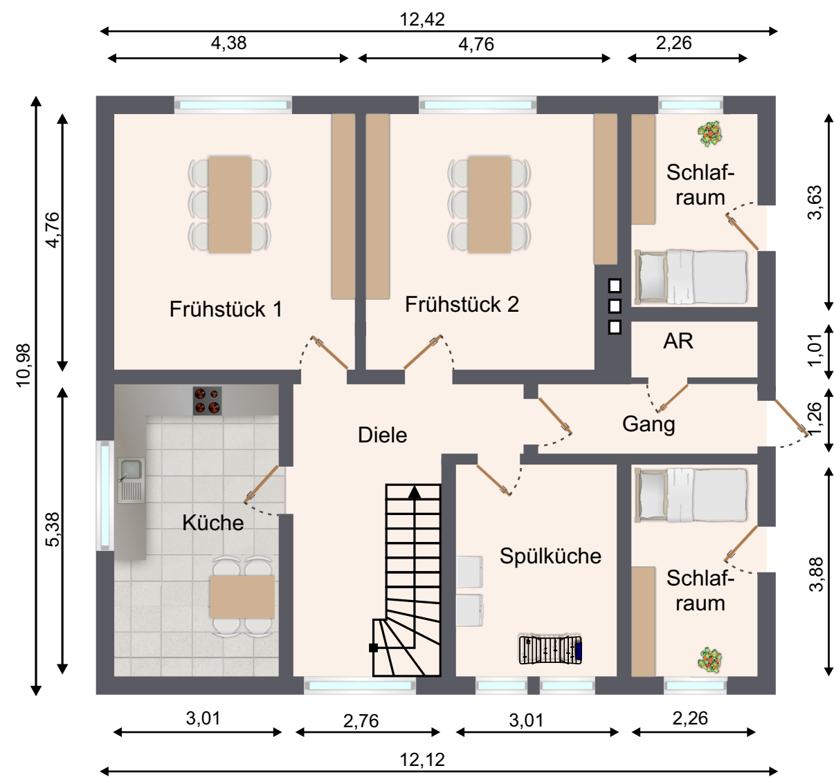
Obergeschoss Anbau
